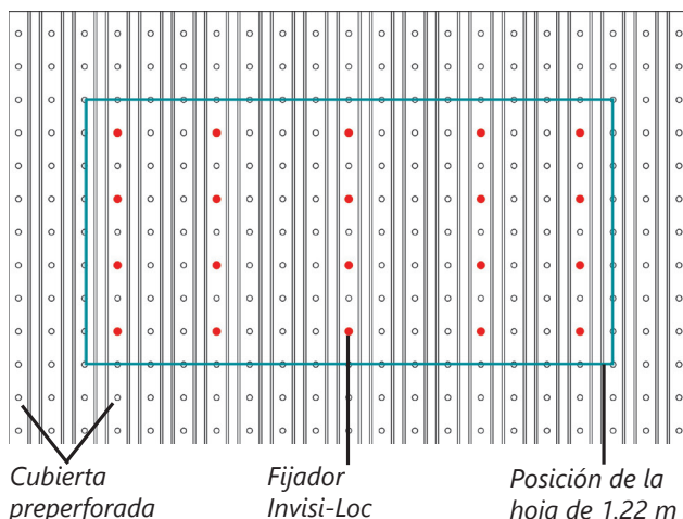
Figura A - Patrón de cuadrícula para estructura acanalada para Invisi-Loc®
