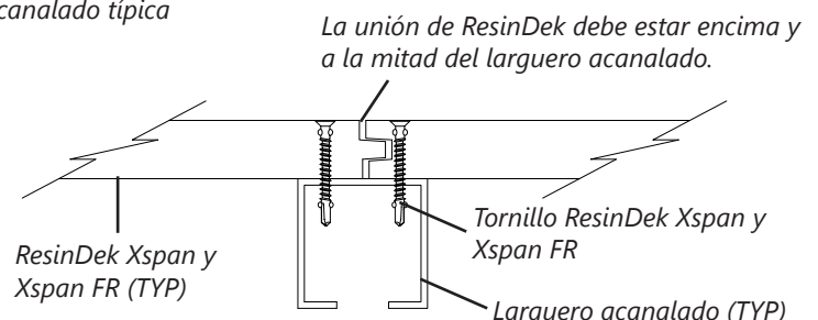
Figura F - Instalación de ResinDek Xspan y Xspan FR en larguero acanalado típica
